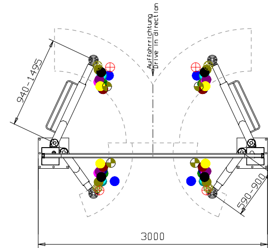
2.30 SL Standardtragarme
