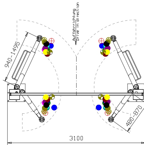
2.30 SL DT mit kurzen 2-fach Teleskoptragarme
